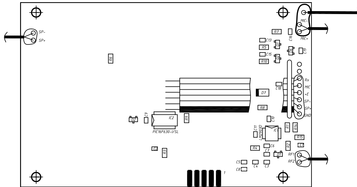
Плата БВД-312R Сборочный чертёж
