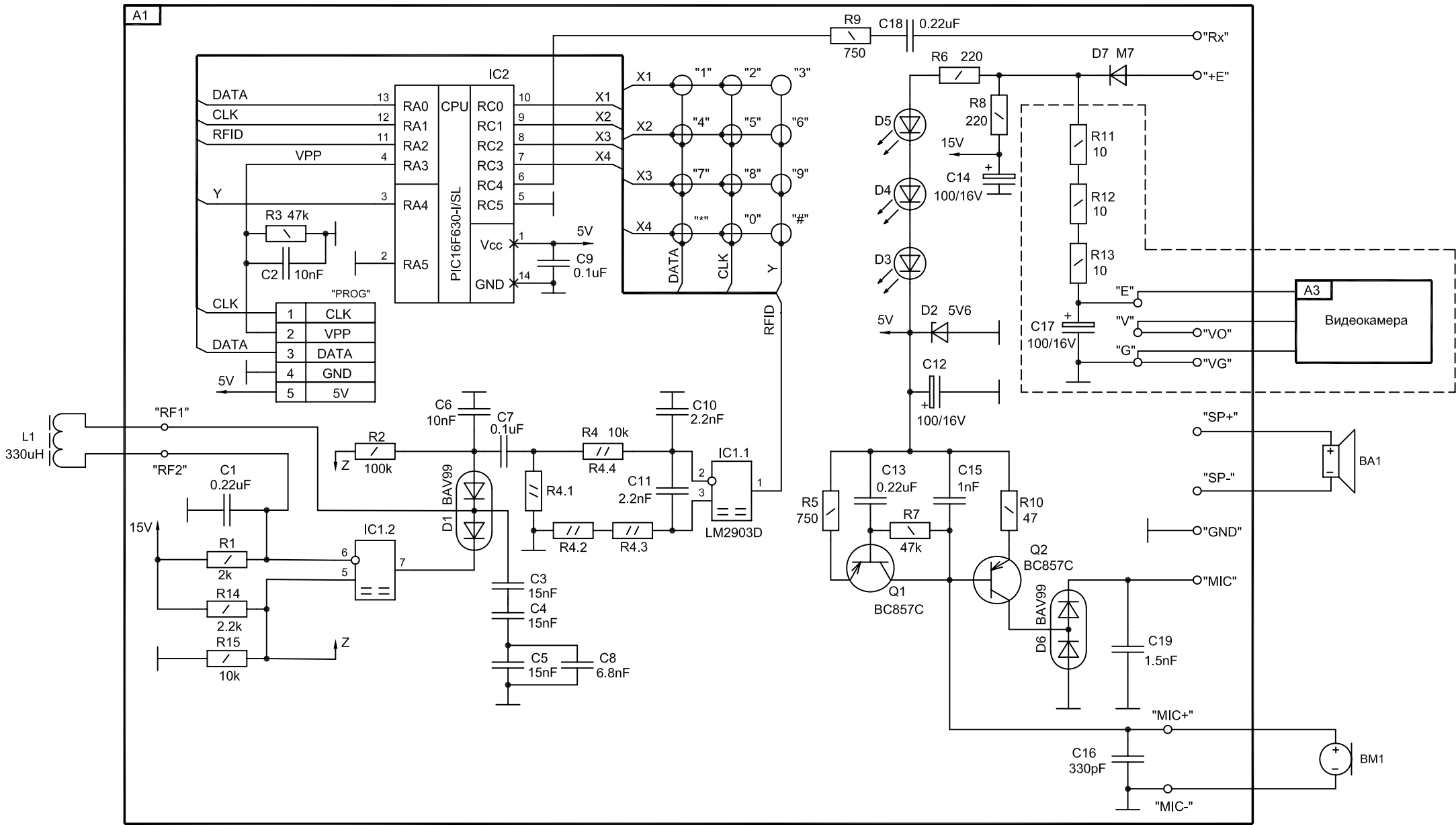
Блок вызова БВД-312 Схема электрическая принципиальная
