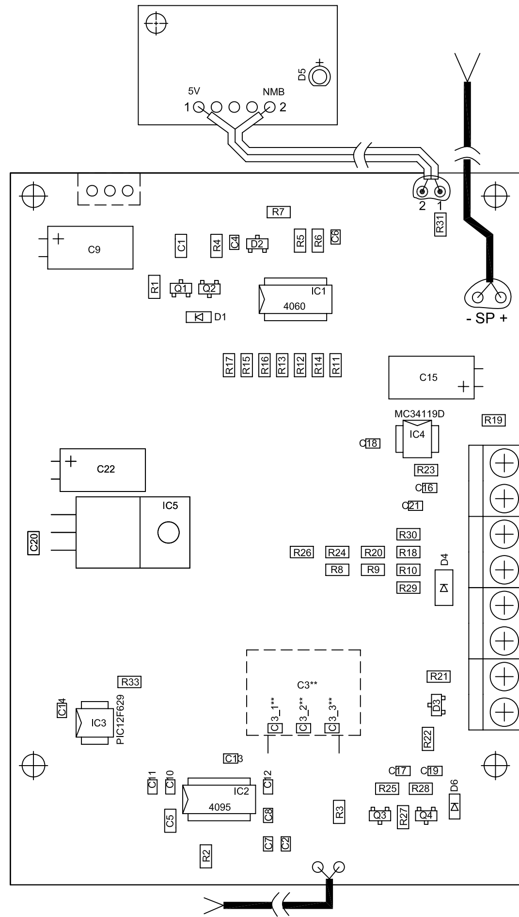
Плата БВД-321RVP Сборочный чертеж
