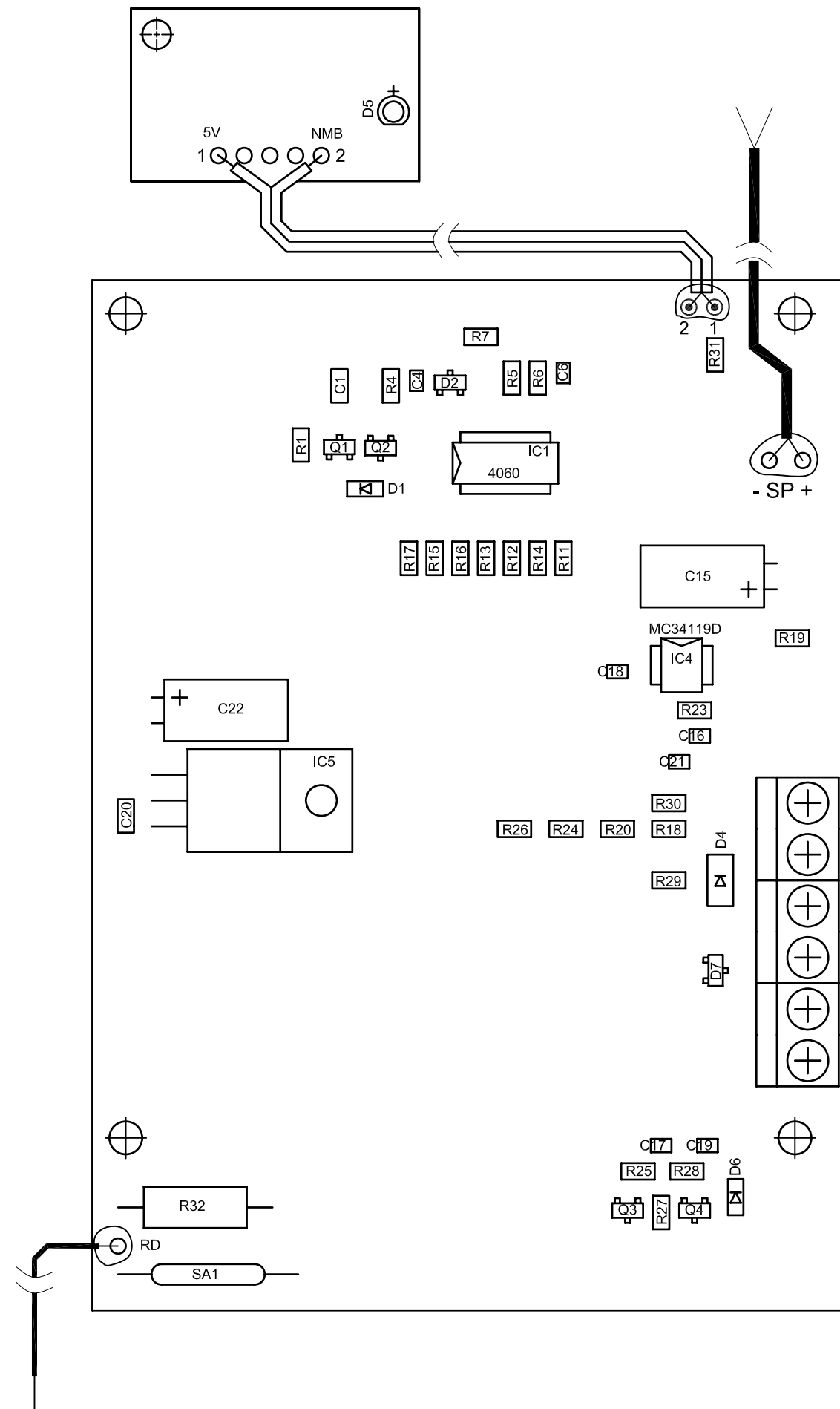
Плата БВД-321 Сборочный чертеж
