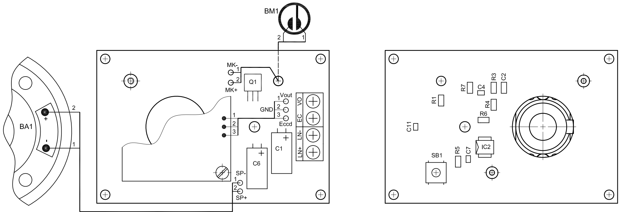
Плата БВД-104СВ
